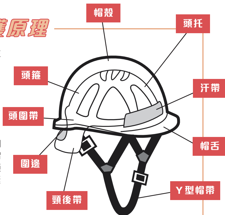
圖一、安全帽的一般設計
